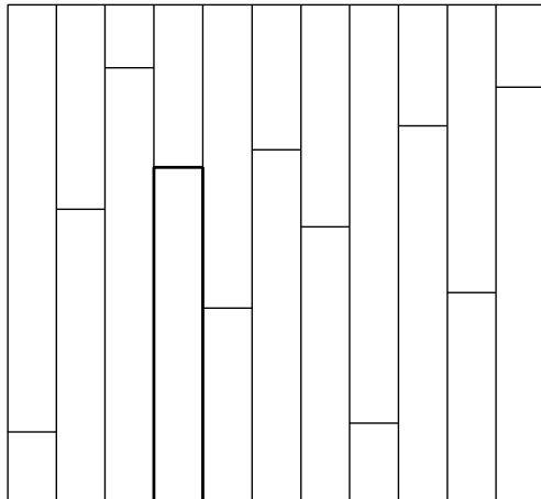
DRP13 Ungeordneter Verband
